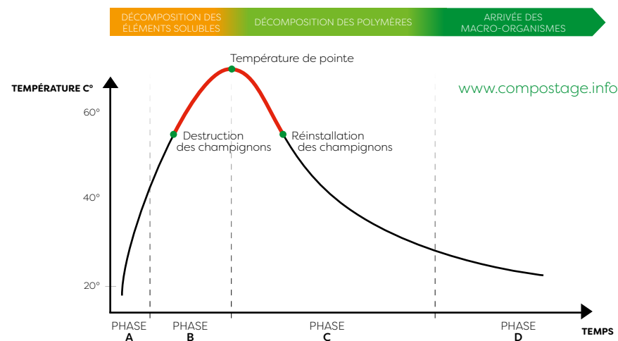
Figure n°2 : ÉVOLUTION DE LA TEMPÉRATURE AU COURS DU COMPOSTAGE D'EFFLUENTS DE FERME.
