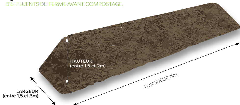
Figure n°4 : SCHÉMA POUR LA MISE EN PLACE DES TAS D'EFFLUENTS DE FERME AVANT COMPOSTAGE.
